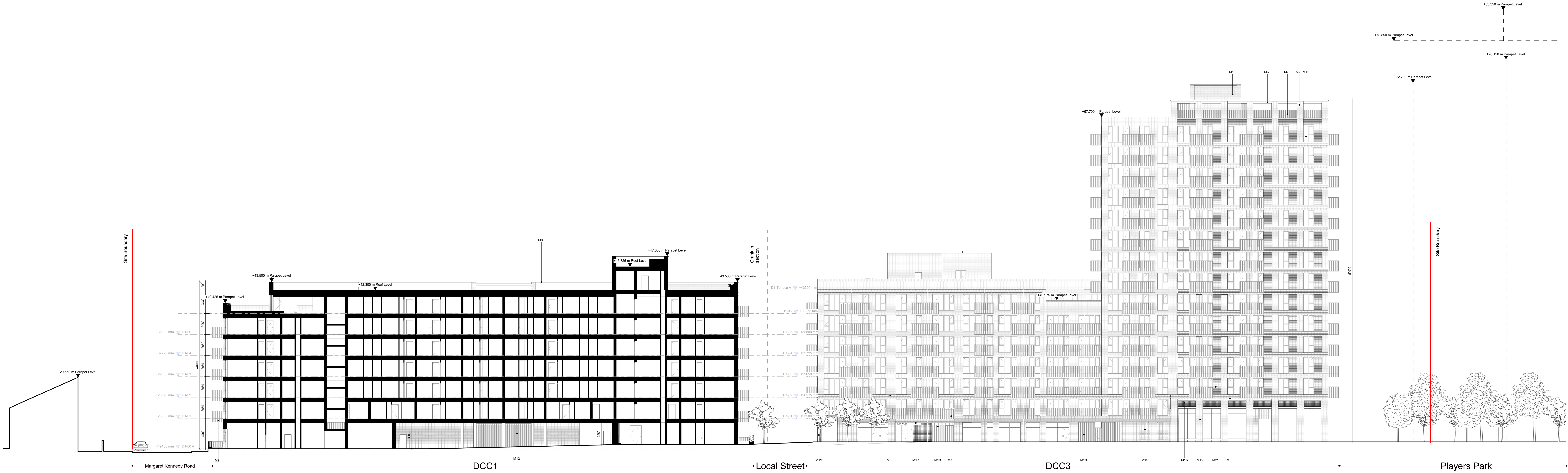
Site Section 3 1:200
